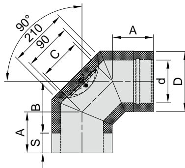
Bogen 90° mit Reinigungsverschluss
