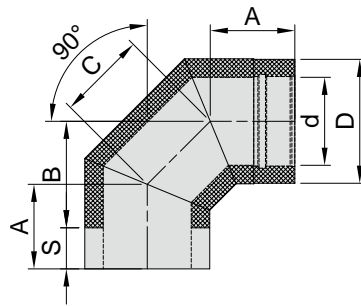
Bogen 90° ohne Reinigungsverschluss
